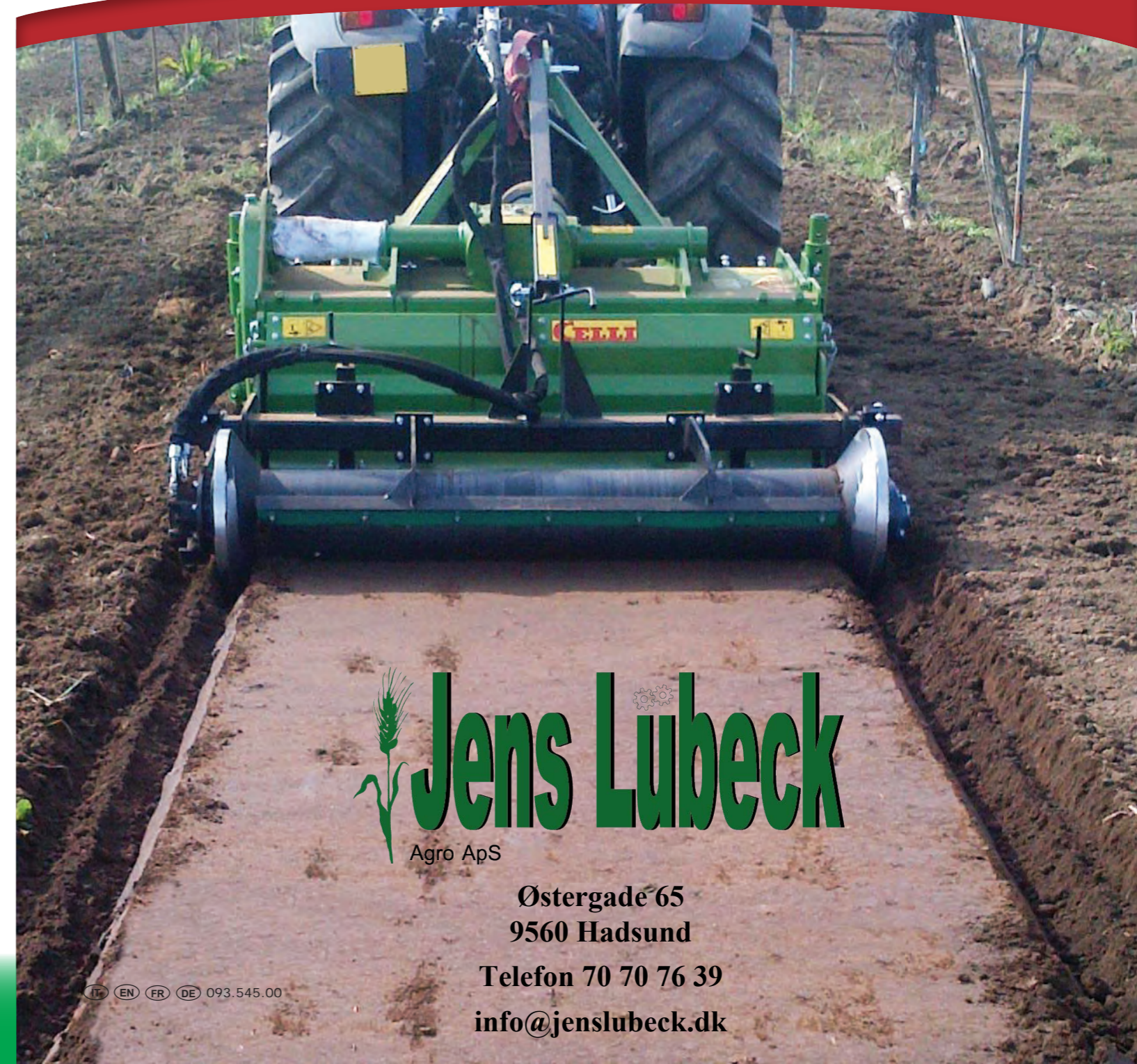
ARES BF con rullo cilindrico baulatore idraulico a richiesta ARES BF with hydraulic roller hydraulic bed former on demand ARES BF avec rouleau hydraulique butteuse hydraulique sur demande ARES BF mit hydraulischer Walze hydraulischer Beetformer auf Anfrage.
